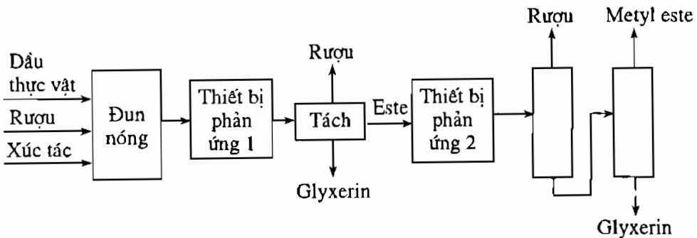
Hình 4.4. Sơ đồ sản xuất biodiesel theo phương pháp liên tục.
