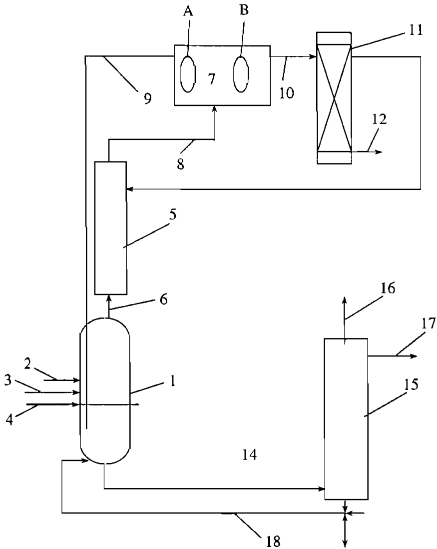
Hình 8.2. Sơ đồ sản xuất etyl lactat liên tục trong công nghiệp:
